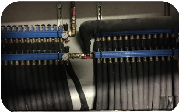
Collecteur de sondes géothermiques
