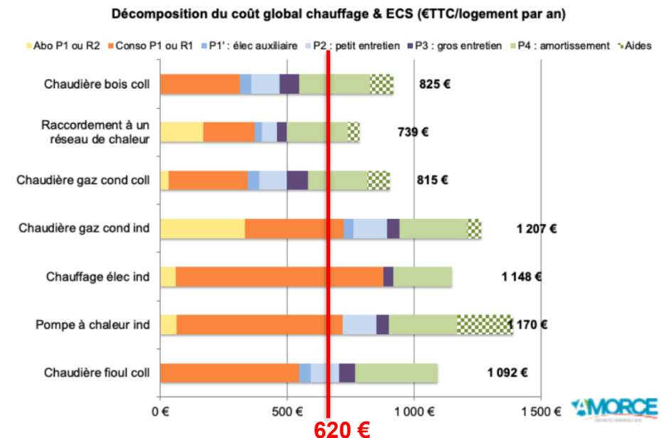
Figure 15 : Décomposition en coût global chauffage et ECS (€TTC/lt/an) pour un bâtiment RT 2012
