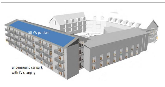
Modélisation d'un immeuble pour retraités avec une installation PV sur le toit et un garage souterrain avec une station de charge de VE à Grafing
