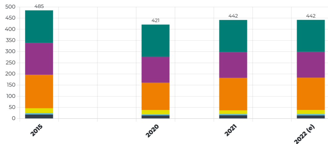
Émissions de gaz à effet de serre de votre territoire par secteur, en milliers de tonnes équivalent CO 2
